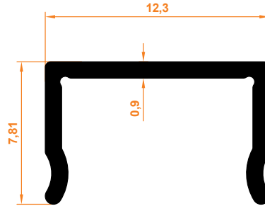
Kare Çita Square Slat
