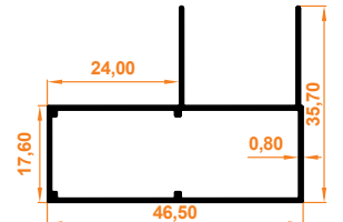
Süper Orta Kasa Profili Super Middle Case Profile
