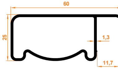
60x25 Yandan Kanallı 60x25 Side Slot
