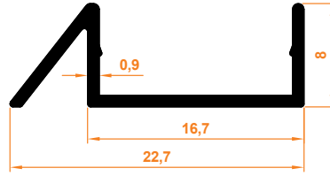
Nobel Eşiksiz Profili
