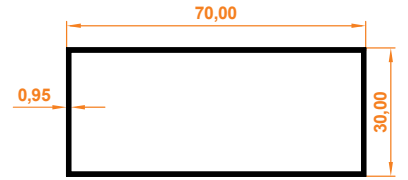
30x70 Kutu Profil 30x70 Box Profile
