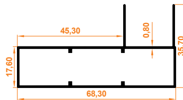
Süper Büyük Kasa Profili Super Big Case Profile
