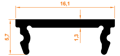
Takviyesiz Cam Tutucu Çita Profil Non-Reinforced Glass Holder Lath Profile
