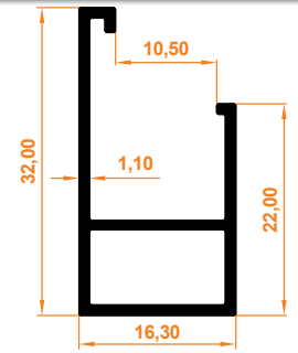
8-10 mm Cam Altı Profil 8-10 mm Glass Bottom
