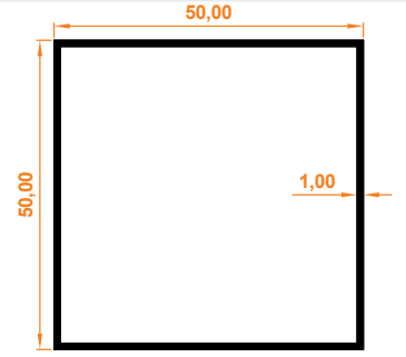
50x50 Kutu Profil 50x50 Box Profile
