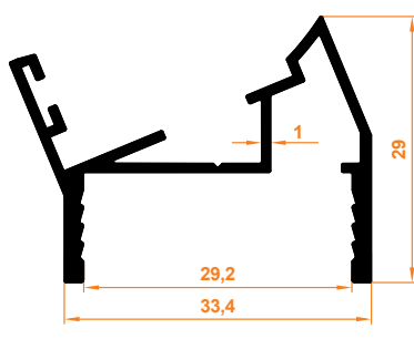
22,5° Dönüş Profil 22,5° Return Profile
