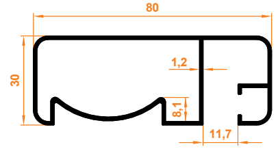
80x30 Yandan Kanallı 80x30 Side Channel
