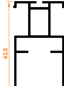
Junior Kanat Profil Junior Wing Profile
