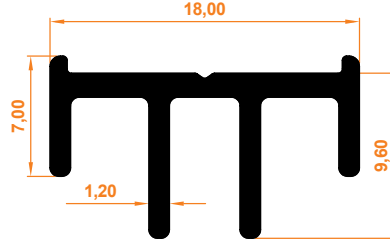
İspanyollet Karşılık Profili Espagnolette Provision Profile
