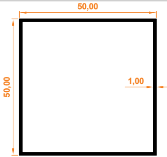
50x50 Kutu Profil 50x50 Box Profile
