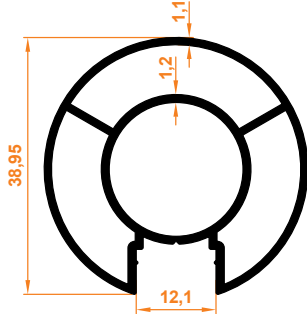
40x1,1 mm Tek Kanallı Çiftli Dikme 40x1,1 mm Single Slot Double Column
