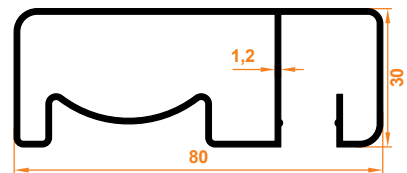
80x30 Yandan Kanallı 80x30 Side Slot
