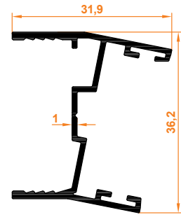
11° Dönüş Profil 11° Return Profile
