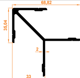
Aldoks (Orta) Köşe Takozu Aldoks (Medium) Corner Wedge
