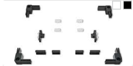
Slım Seri İçten Gergi Aksesuar Seti Slim Serie Internal Tensioner Accessory Set
