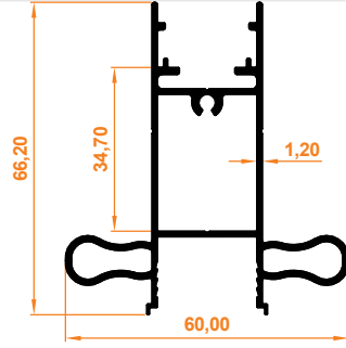
İspanyollet Çekme Kol Profili Espagnolette Pull Handle Profile
