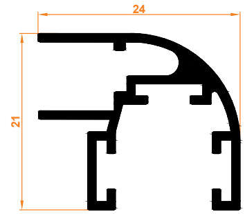
Köşe Dönüş Fitol Corner Return Wick
