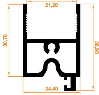
Sabit Panel Açılır Alt Baza Profil Fixed Panel Pop-up Base Profile
