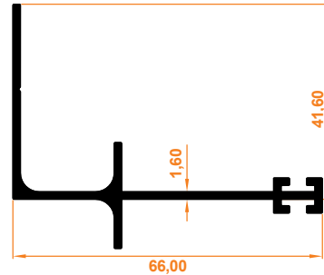
Açılımsız Çift Fıtil Yan Ray L Kasa Profil Double Weatherstrips Without Opening Side L Case Profil
