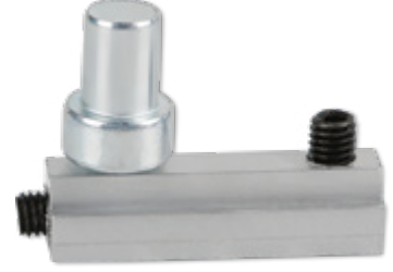
Menteşe Takımı Pim Ayarlı Alt Hinge Bottom - Adjustable
