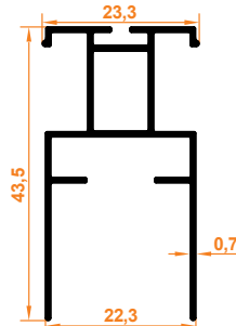
Junior Kanat Profil
