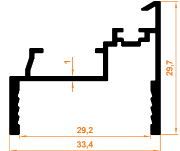
Sabit Cam Kilit Karşılığı Profili Stable Glass Lock Prevention Profile
