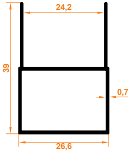
Junior Kasa Profil
